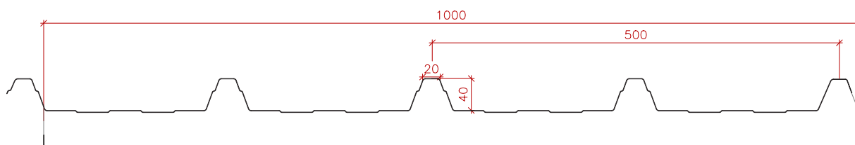
Sección transversal - Cross section
