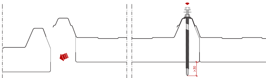
Detalle de Encaje - Joint Detail
