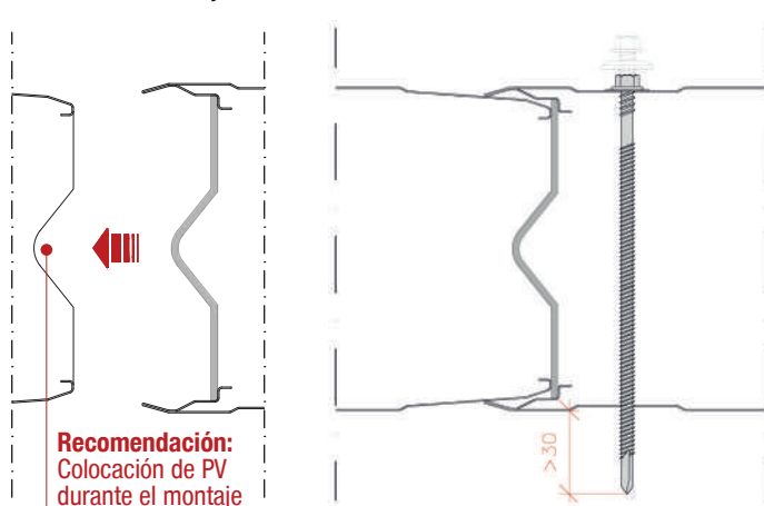
Detalle de Encaje - Joint Detail
