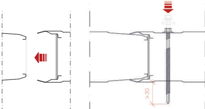
Detalle de Encaje - Joint Detail
