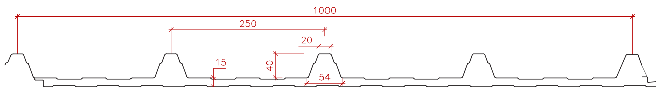
Sección transversal - Cross section
